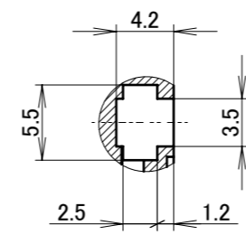
M3ナットスロット_Nut Slot (2:1)
